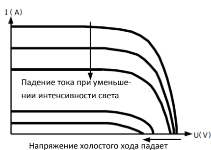
Рисунок 1-3. Зависимость выходных параметров модуля от освещенности
